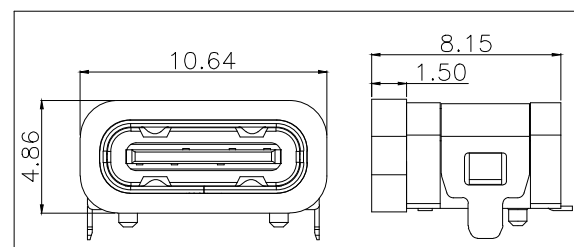
加防水圈示意图
